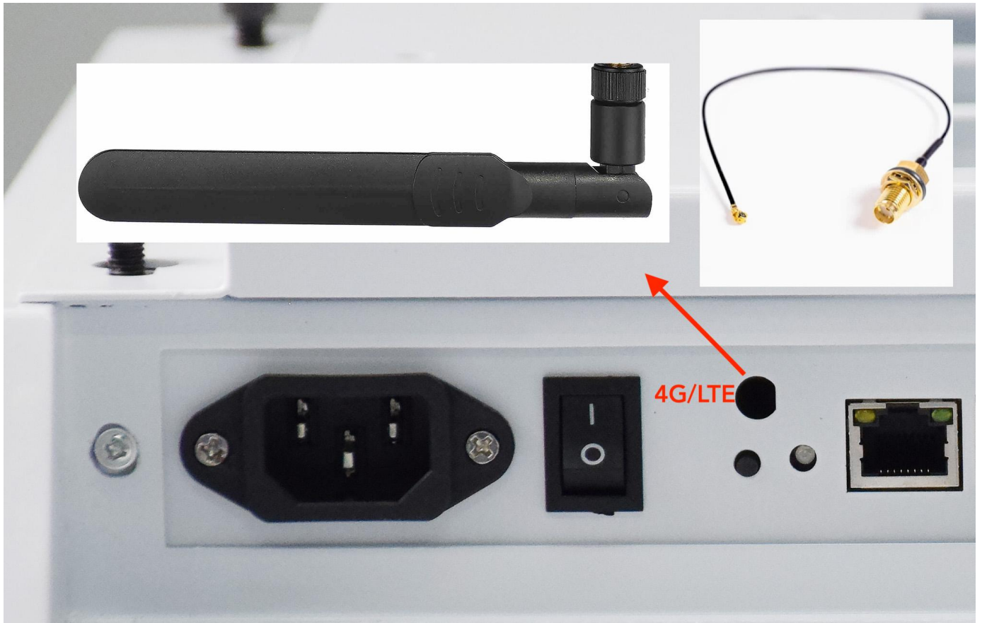
4G Antenna
